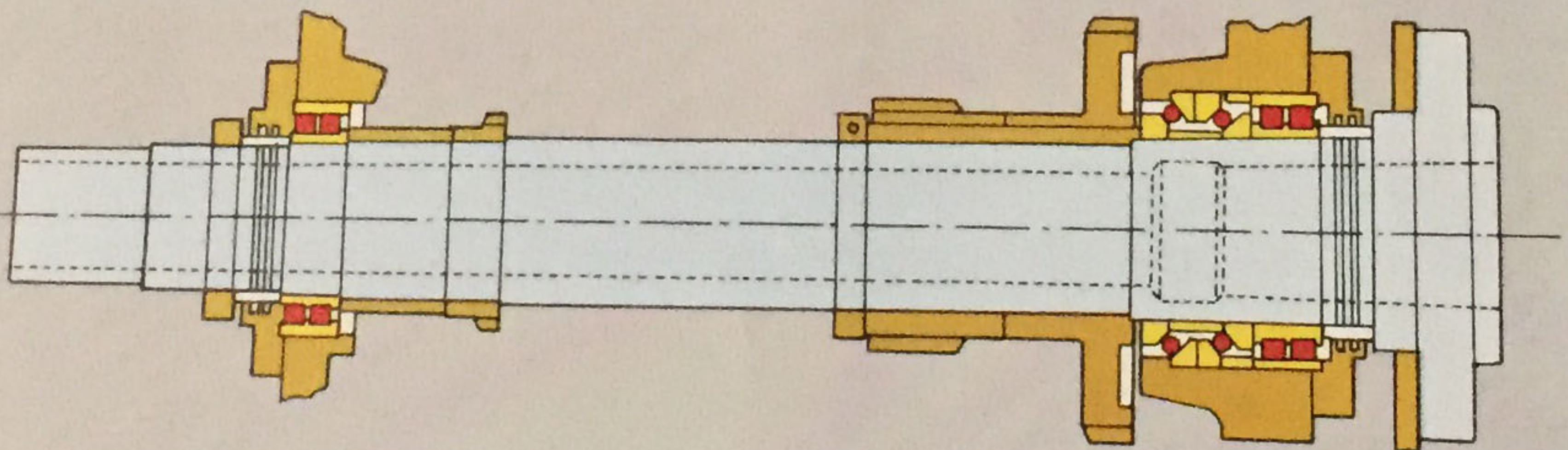
Hauptspindel-Lagerung (MD 22 S)
